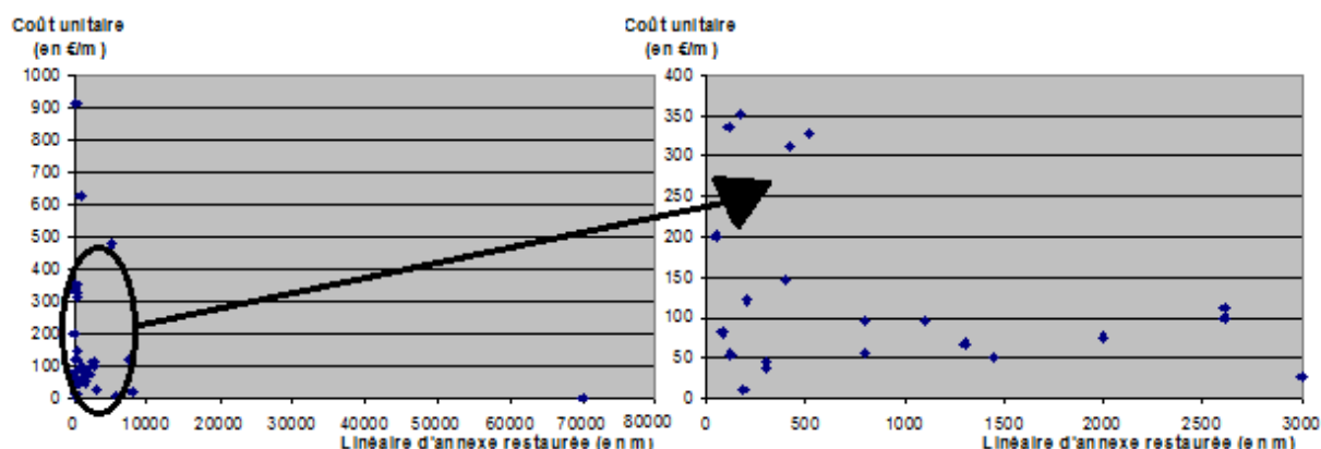
Graphique des coûts unitaires (en €/m d'annexe restaurée) en fonction du linéaire d'annexe restaurée (en m)
