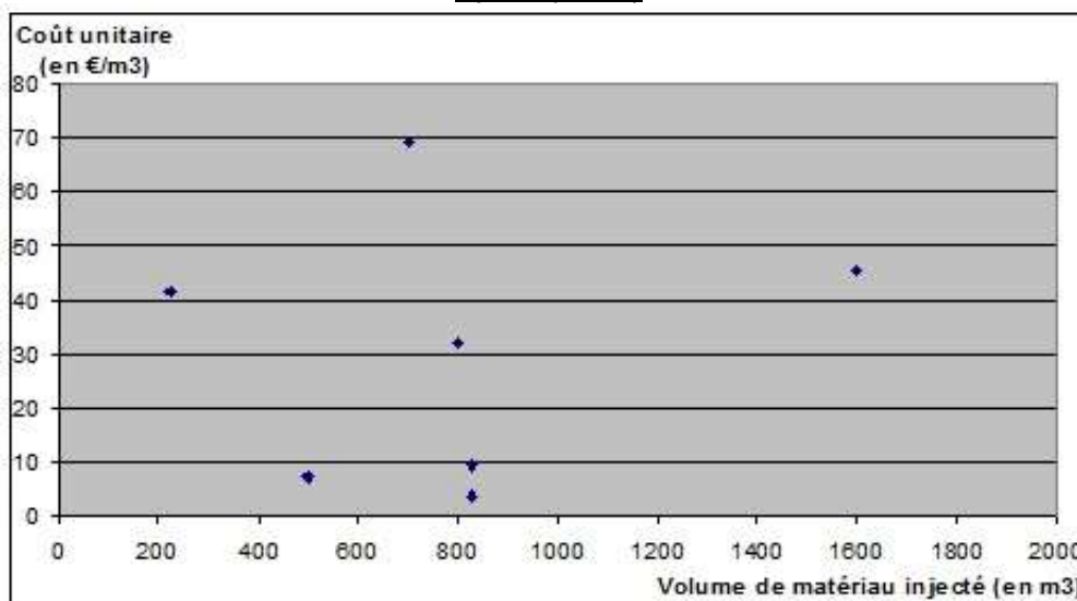
Graphique des coûts unitaires (en €/m 3 de matériaux injectés) en fonction du volume de matériau injecté (en m 3 )
